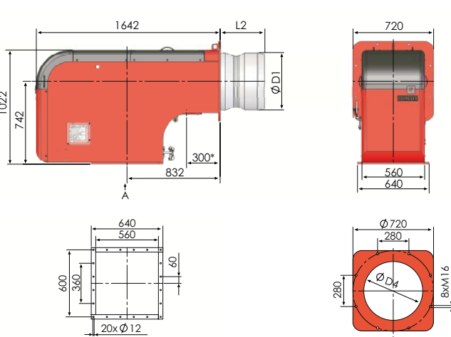
ВИД А Монтажный фланец воздушного канала
