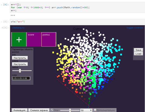
Рис. 3. Пример визуализации в блокноте, созданной с помощью визуального языка.
