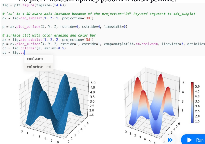
Рис. 2. Код визуализации и результат его работы.
