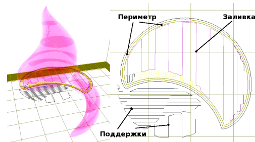
Рис. 6. Слой, получившийся в результате слайсинга.
