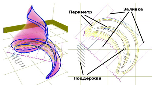
Рис. 7. Пример некорректного формирования слоёв вследствие ошибок модели.
