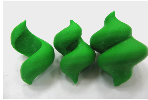
Рис. 5. Множества G(T) для T = 2\pi/\alpha , 3\pi/\alpha , 4\pi/\alpha .
