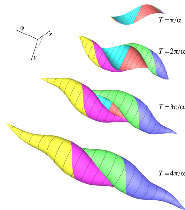
Рис. 2. Развитие множества достижимости G(T) .
