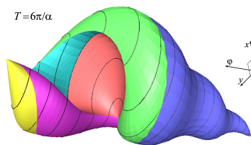
Рис. 3. Множество достижимости G(T) для T = 6\pi/\alpha при несимметричном ограничении u \in [-1, +0.25] .
